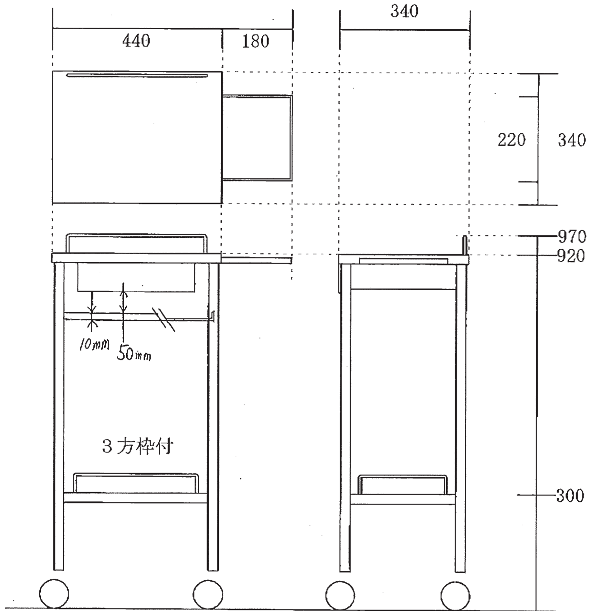
キャスターφ75対角ストッパー付
