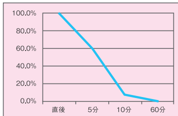
大腸菌
