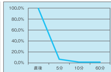
サルモネラ
