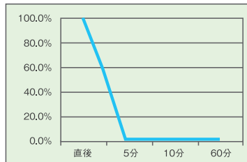
緑膿菌
