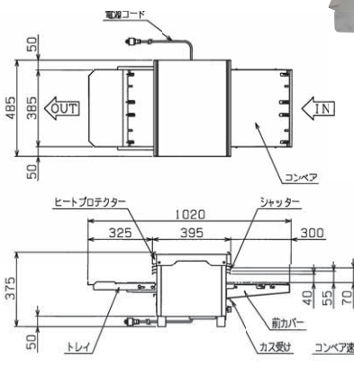
■ コンベアオープン(焼物用)仕様表
