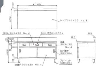
BHD-156N
