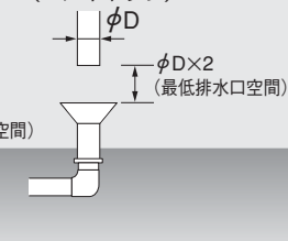
■スカッパー方式 (エアギャップ)
