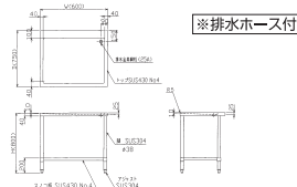
■水切台 (バックガードなし)
