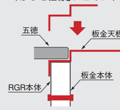
■ガスレンジ+板金製品の「かぶせ仕様」ジョイント
