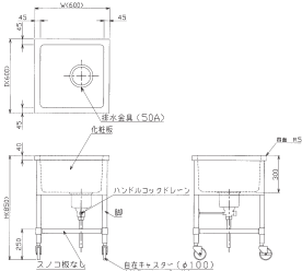
BMS-066
