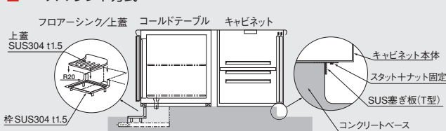
■ベースマウント方式
