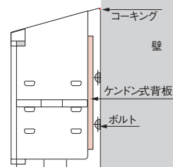
取付方法
