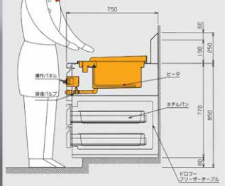
配置 B-B
