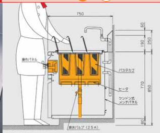
配置 D-D
