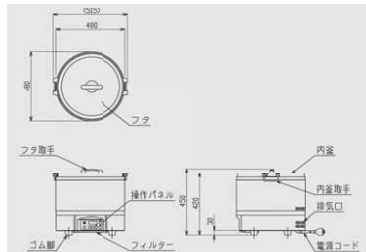
■三面図
