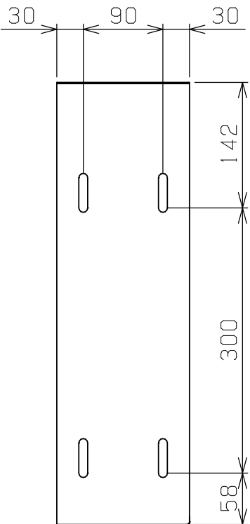
側面
