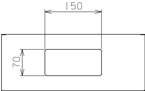
背面
