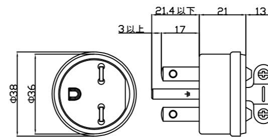
単相200Vプラグ形状 (接地極付 15A 250V)
