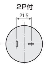
JIS 2極差込接続器 20A 250V
