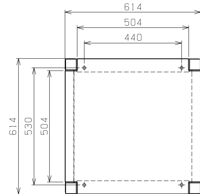
矢視A-A
