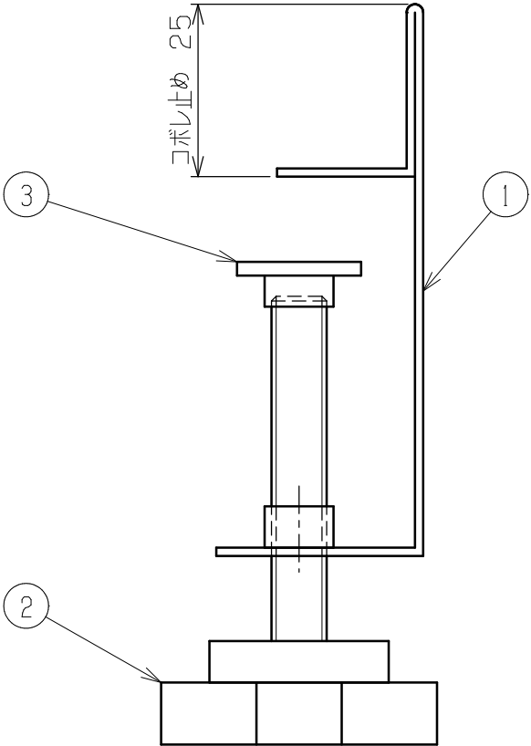
部品取付詳細 (S = 1 : 1)
