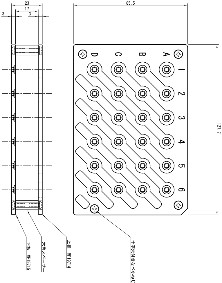
組立図
