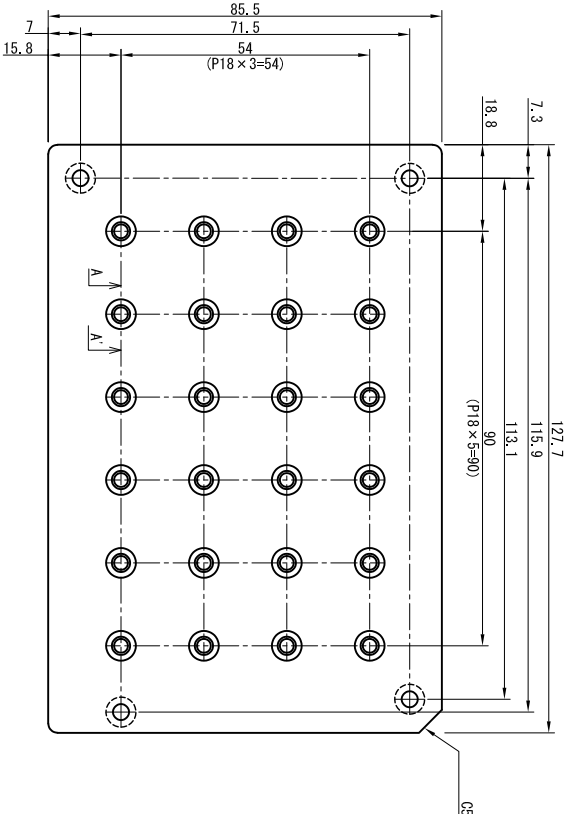
下板寸法図
