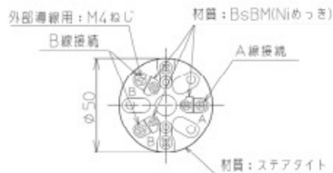
端子板
