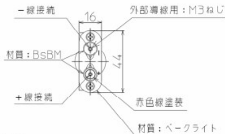
端子板
