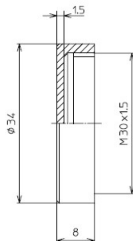
4. FL-PA30W外形図
