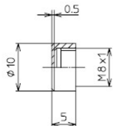
2. FL-PA12W外形図
