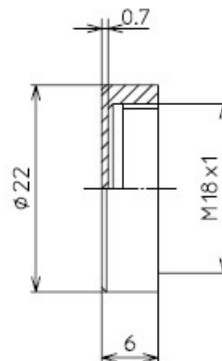
3. FL-PA18W外形図
