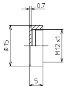
2. FL-PA12W外形図
