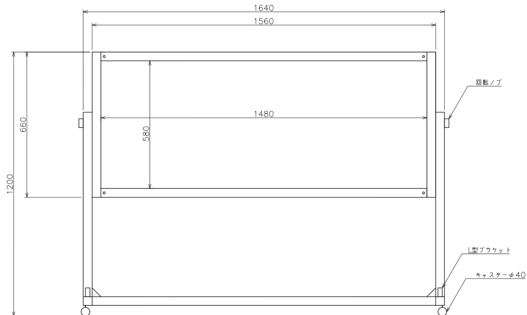
正面図
