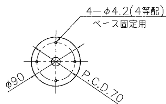
A-A 断面図 取付ベース
