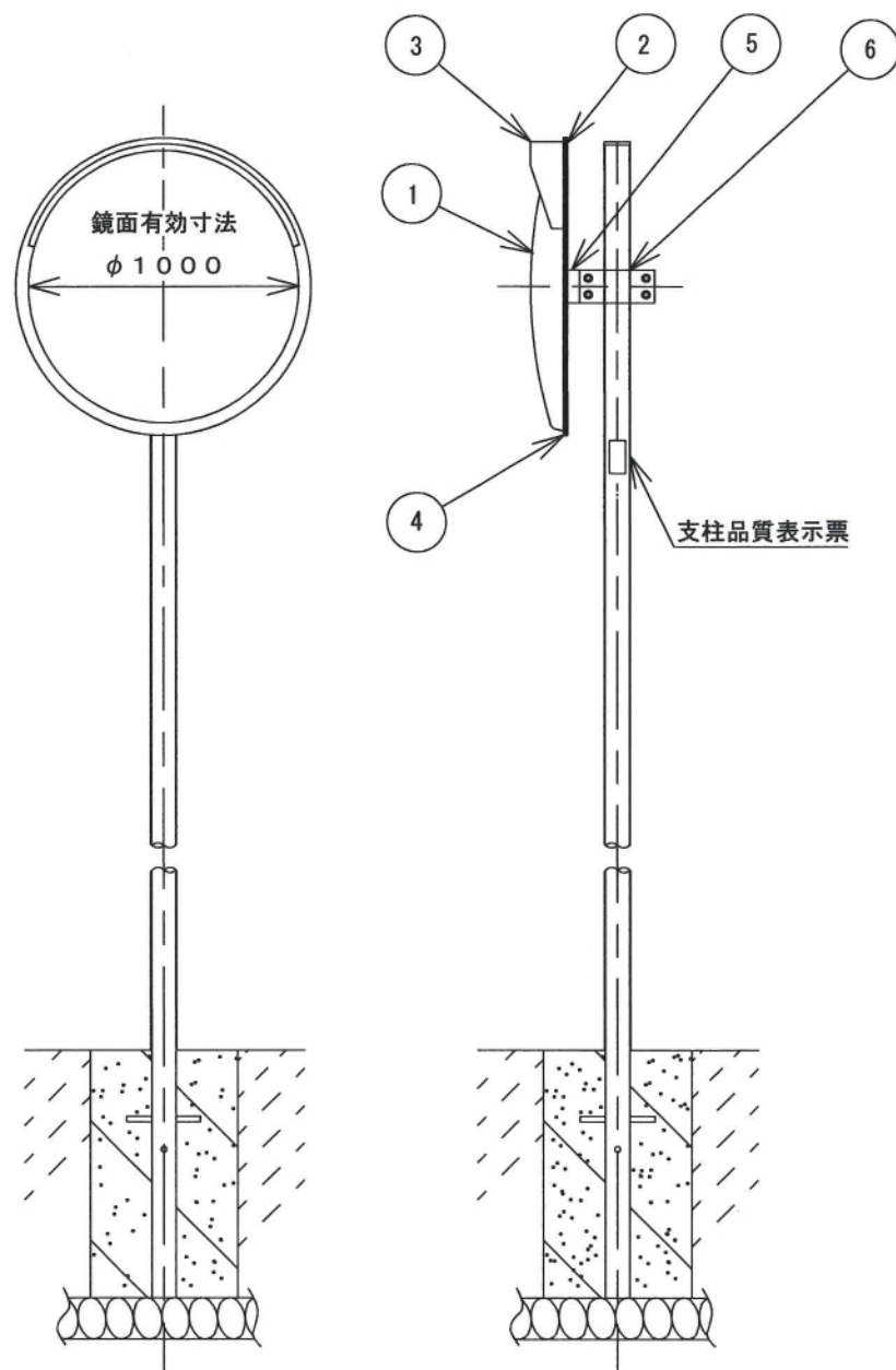
正 面 图
