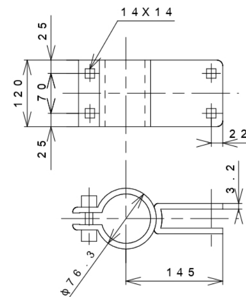
6 . 取付金具
