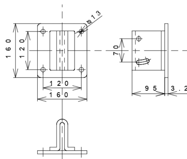
5 . 取付金具
