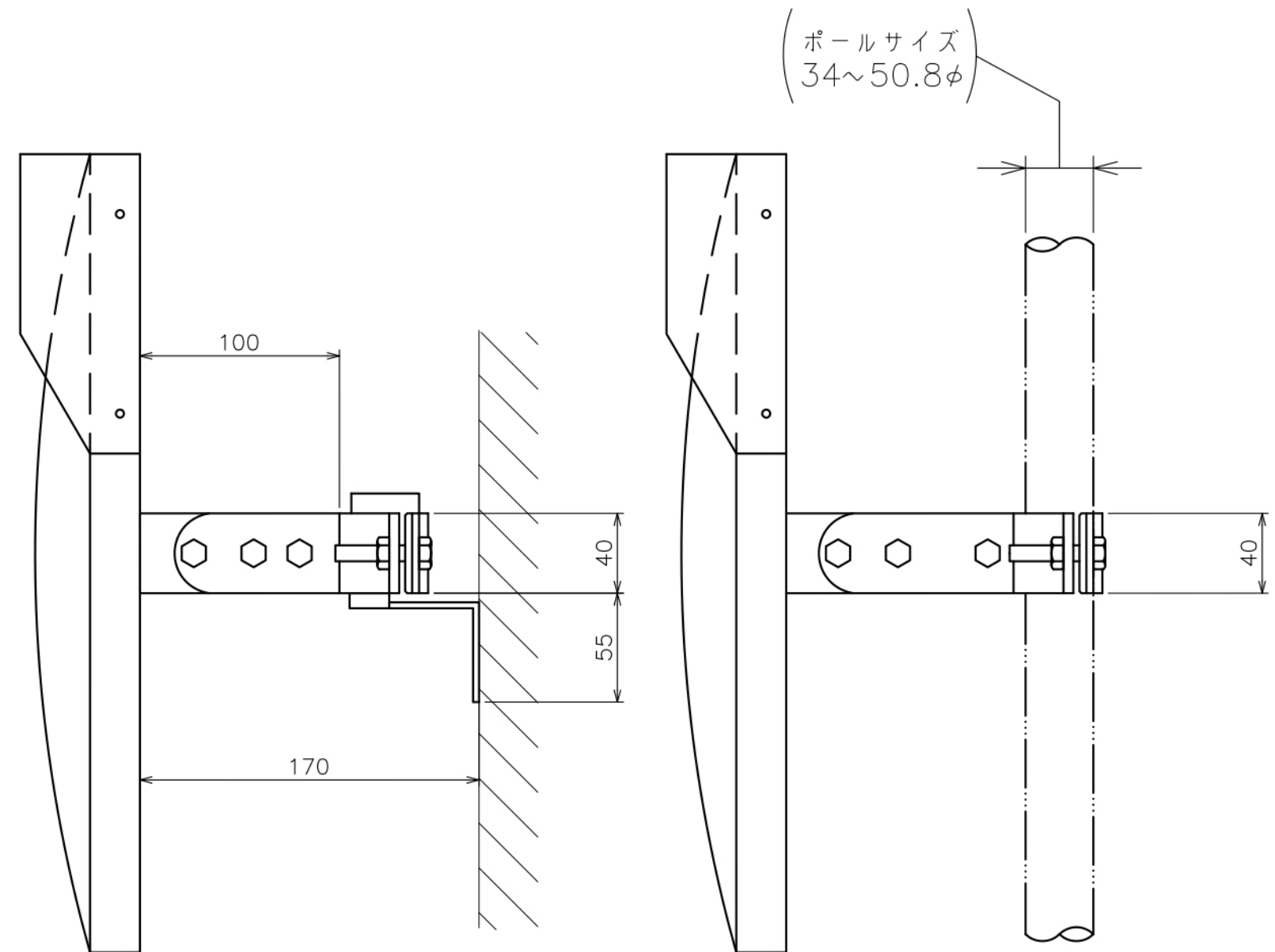
側面図
