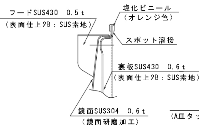
No.3金具 (壁面用金具) S=1:5
