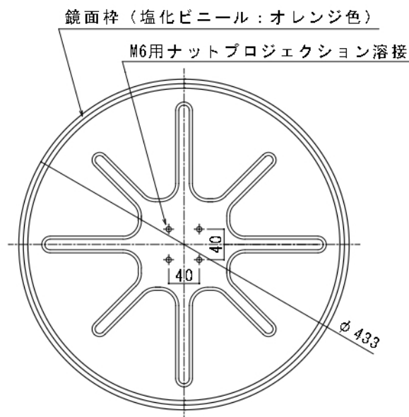
背面図 (S=1:7 裏板 : SUS430 プレス成型)
