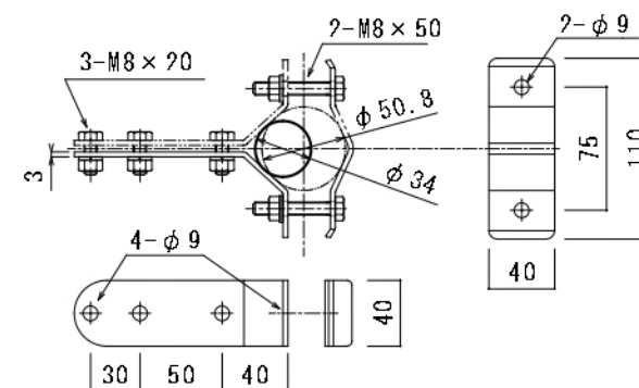
No.2金具 (支柱用金具 : 34φ~50.8φ対応) S=1:5
