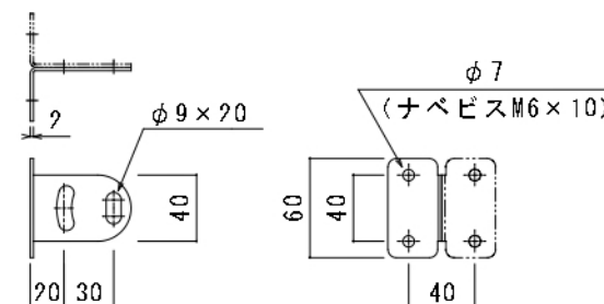
No.1金具 (裏板金具) S=1:5
