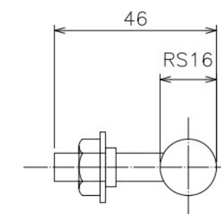
ピボット（ステンレス製）D S=1:1.5
