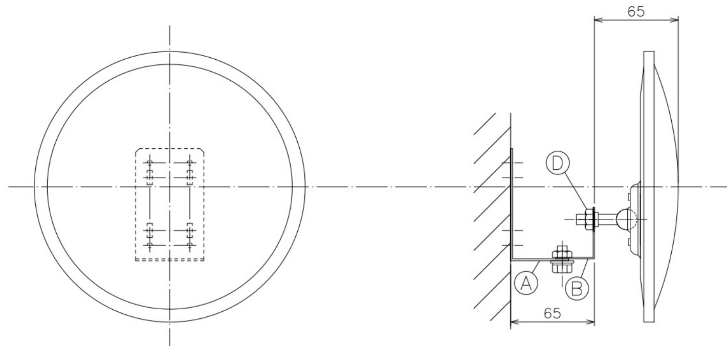
壁取付図
