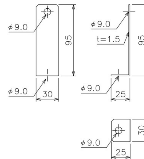
ピボット（ステンレス製）D S=1:1.5
