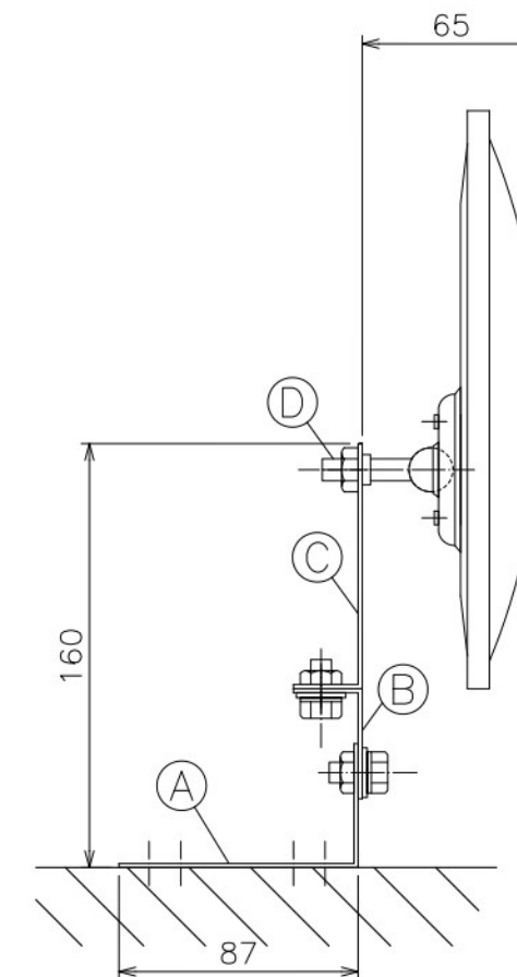
ピボット（ステンレス製）D S=1:1.5
