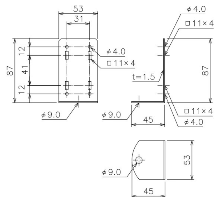
取付ブラケット A
