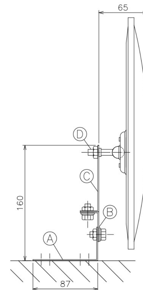
ピボット (ステンレス製) D S=1:1.5
