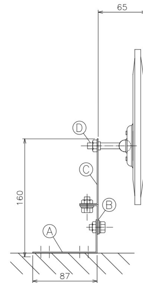
ピボット (ステンレス製) D S=1:1.5
