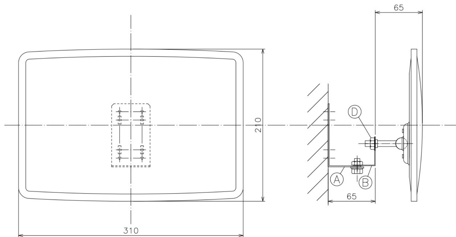
補助ステー B
