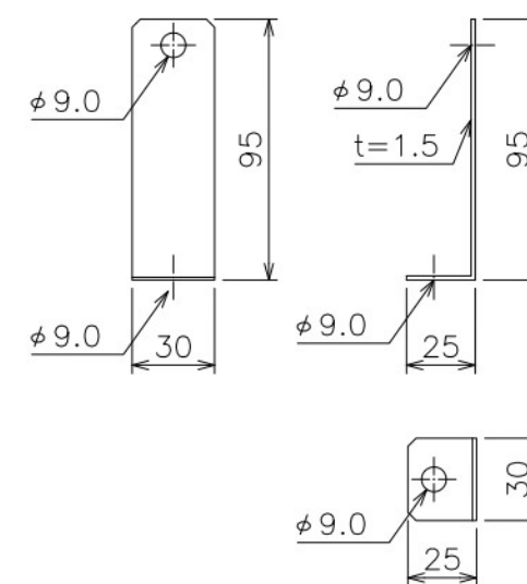
補助ステー C
