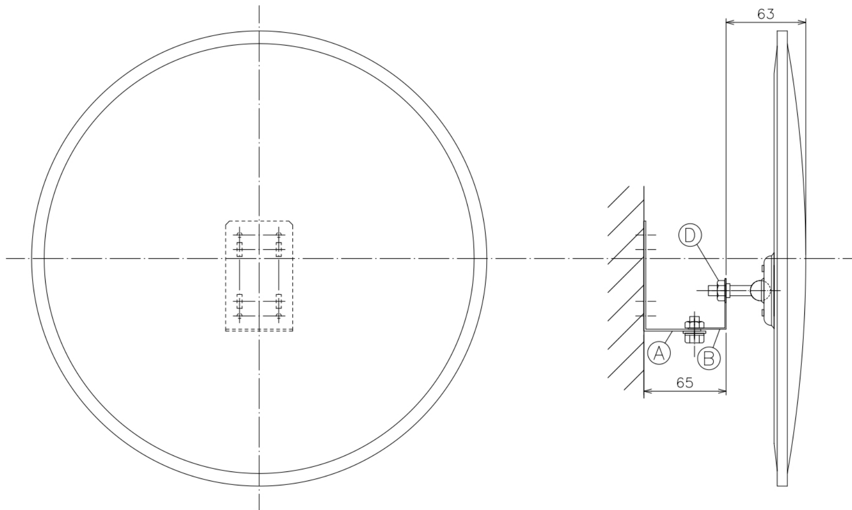
補助ステー B
