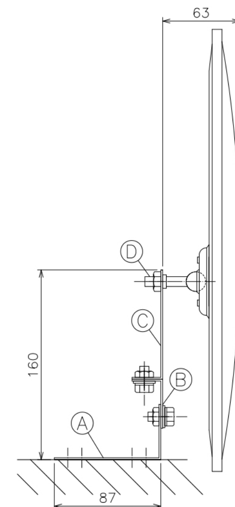
ピボット（ステンレス製）D S=1:1.5
