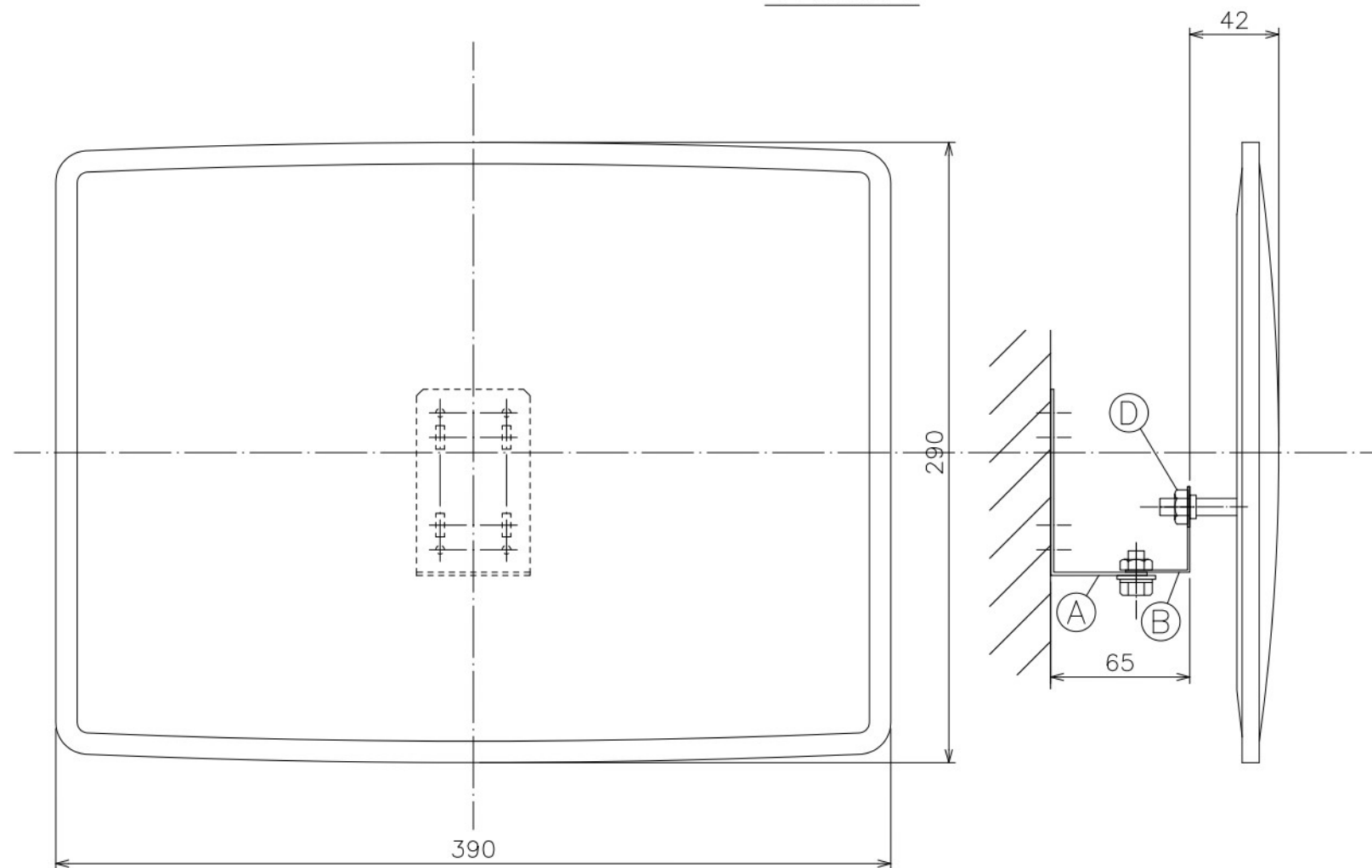
補助ステーB
