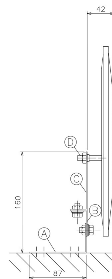
ピボット（ステンレス製）D S=1:1.5
