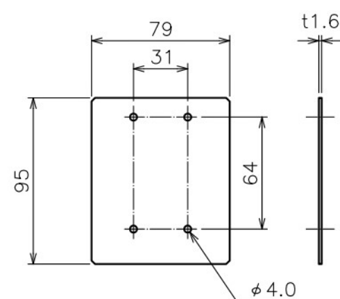
フェンス用挟み込み金具 ①
