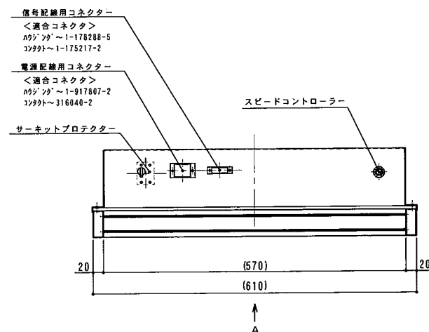
A 矢視図 (S=1/7)
