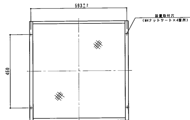
A 矢視図 (S=1/7)
