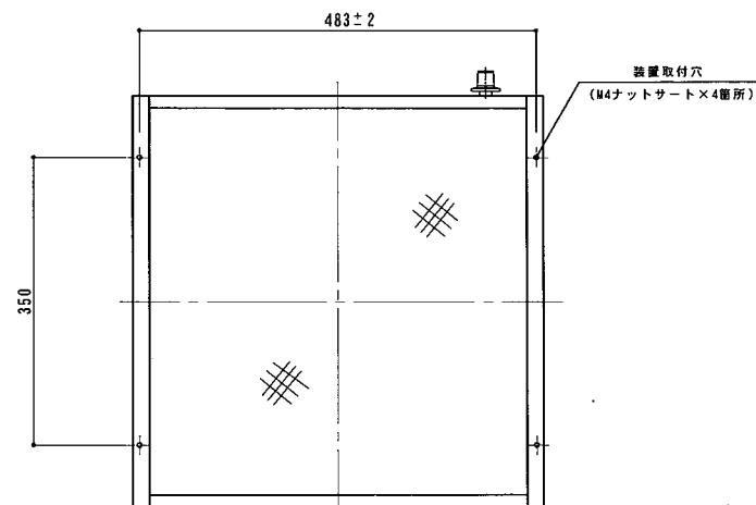
A 矢視図
