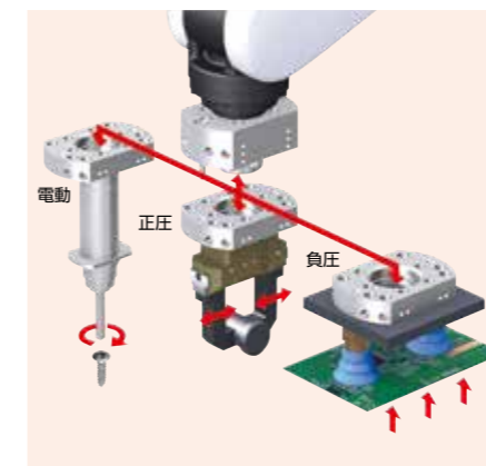
ツールチェンジャー
