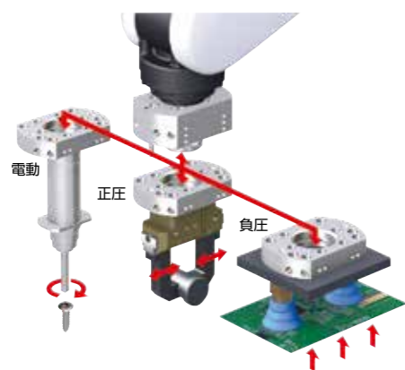
正圧、負圧、電動に対応
