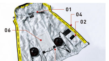
ケーブルストッパー (面ファスナー止め)
