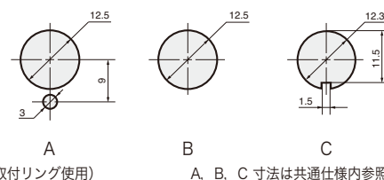
取付寸法図・取付パネル有効板厚
