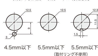
取付寸法図・取付パネル有効板厚
