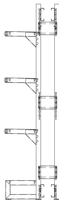
連結部の取付断面図
