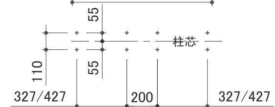
複式アンカー位置 (下穴径φ8.5)
