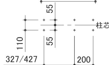
単式アンカー位置 (下穴径φ8.5)
