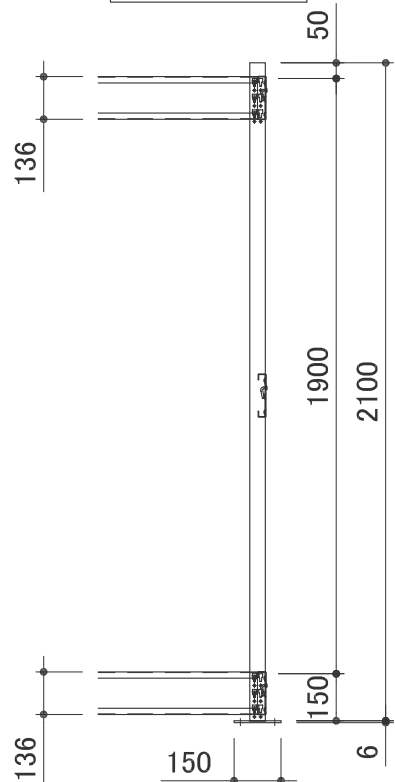
支柱の背面側
