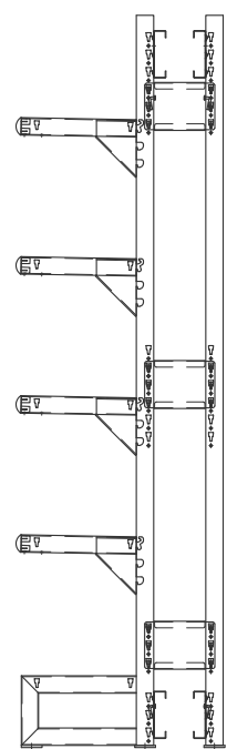
連結部の取付断面図
