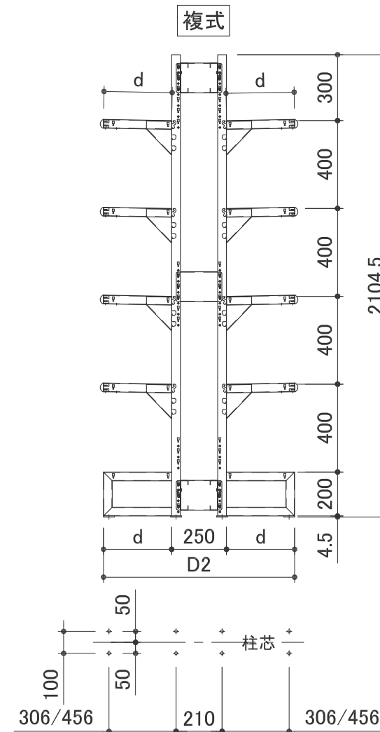
複式アンカー位置 (下穴径φ8.5)
