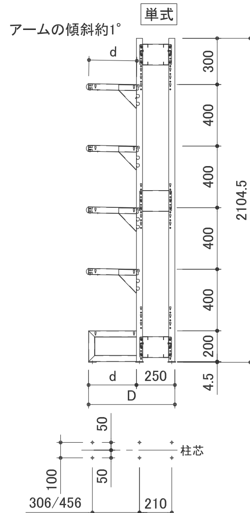
単式アンカー位置 (下穴径φ8.5)
