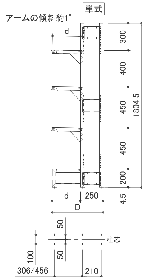
単式アンカー位置（下穴径φ8.5）
