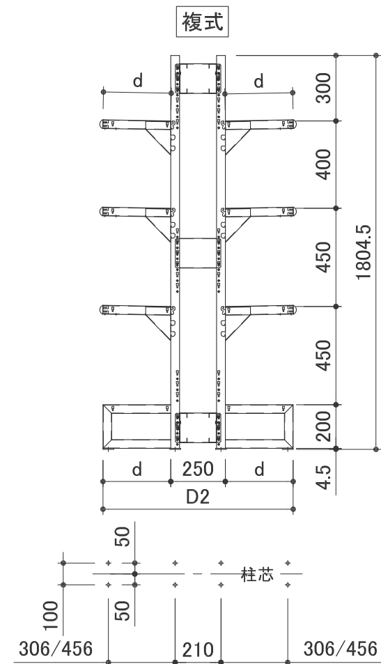
複式アンカー位置（下穴径φ8.5）
