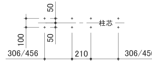
複式アンカー位置 (下穴径φ8.5)
