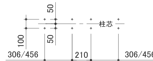
複式アンカー位置（下穴径φ8.5）
