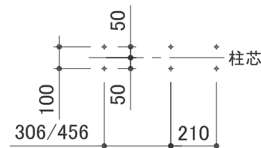
単式アンカー位置（下穴径φ8.5）
