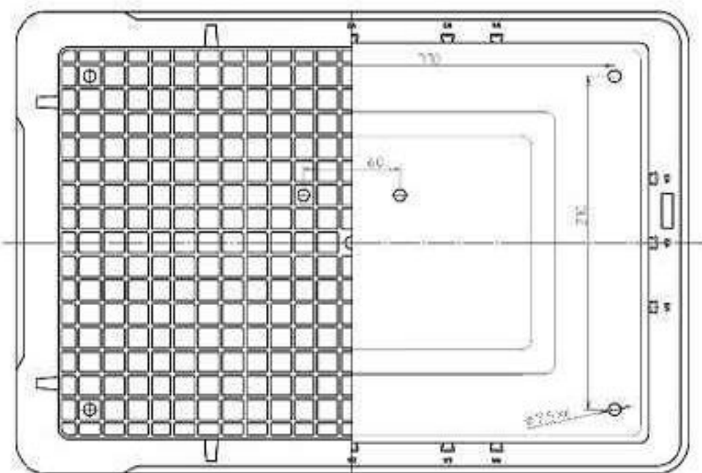
下面図
