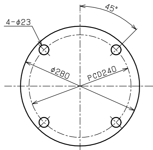
JIS10K 150Aに準用 取付座詳細
