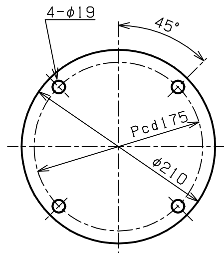
JIS10K 100Aに準用 取付座詳細
