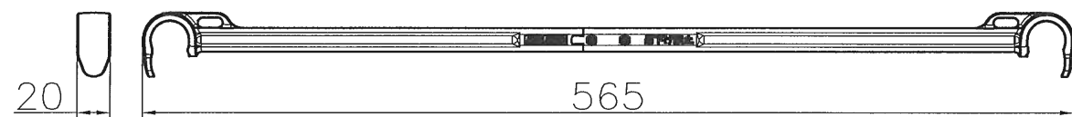
サポートバー（組立図）（2セット入り）
