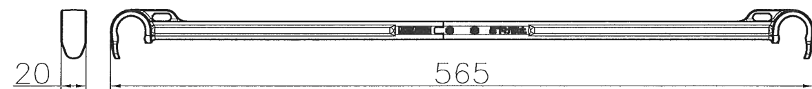
サポートバー（組立図）
