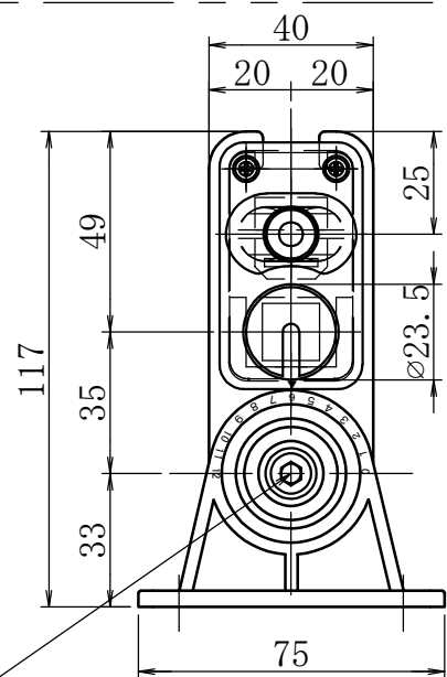
取付ホルダ(付属品)
