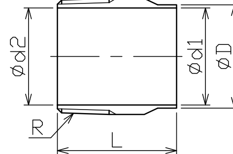
外形形状 タイプ 5
