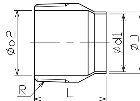
外形形状 タイプ 5
