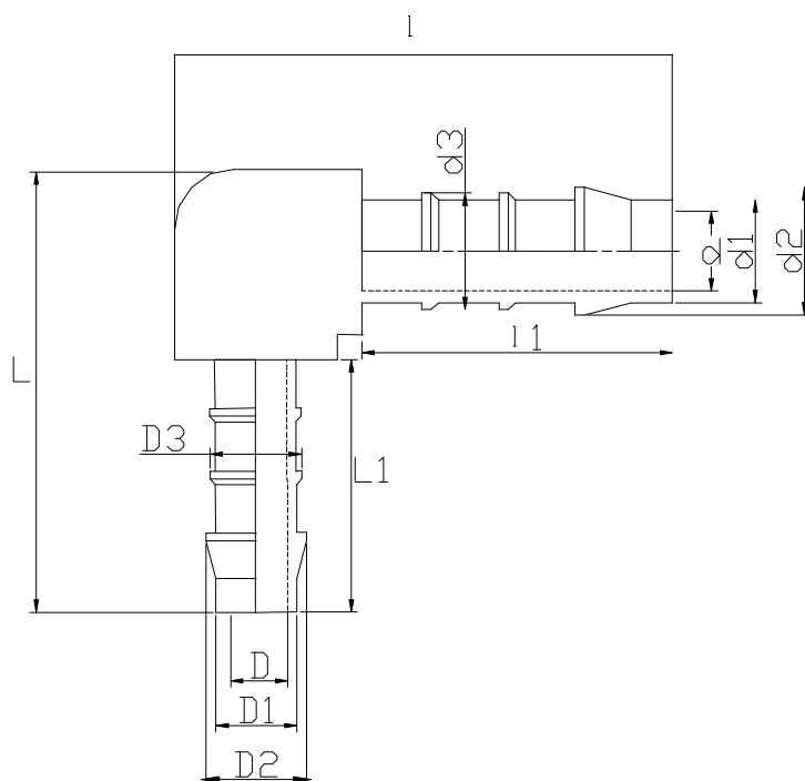
異径ユニオンエルボ
