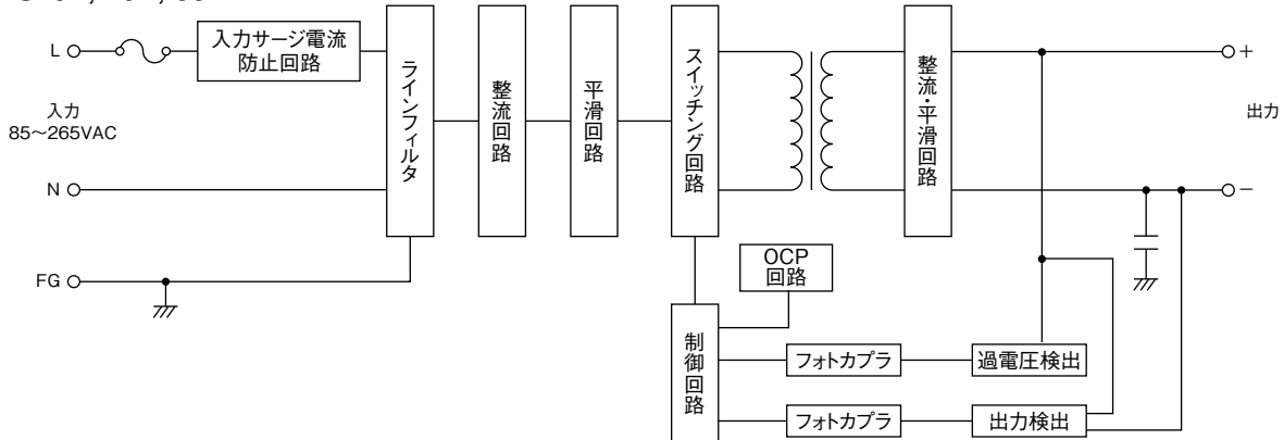
ZWS50B, 75B
