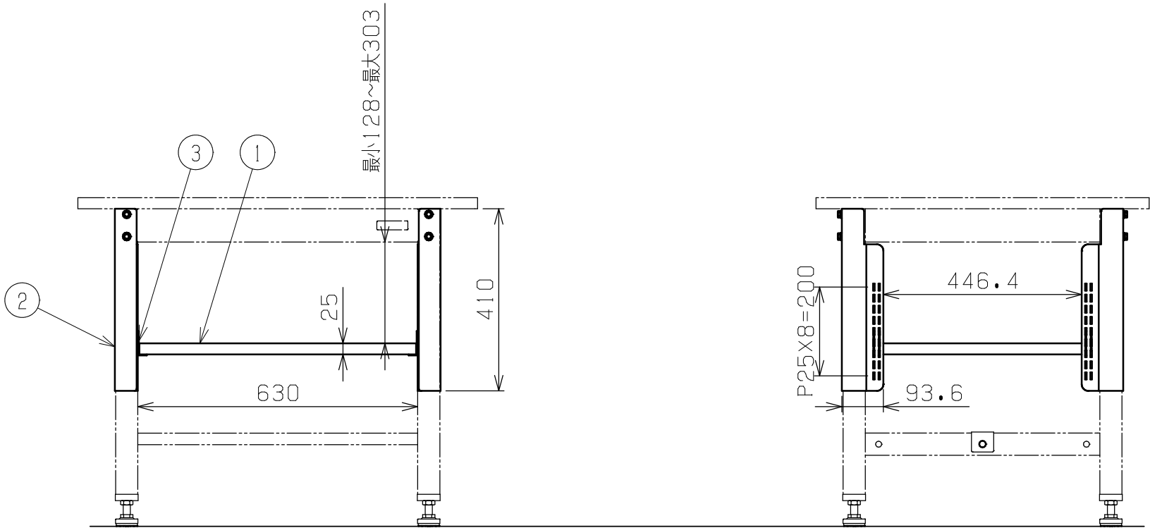
〈中棚取付例〉
