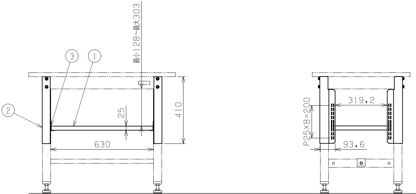
〈中棚取付例〉
