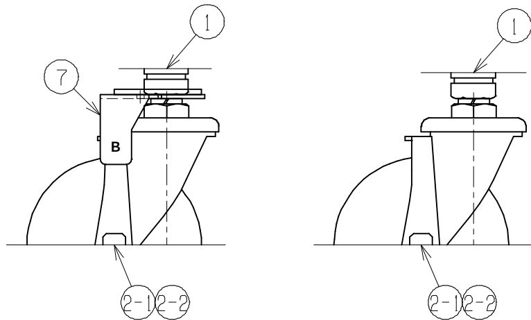
キャスター取付部詳細 尺度1:3
