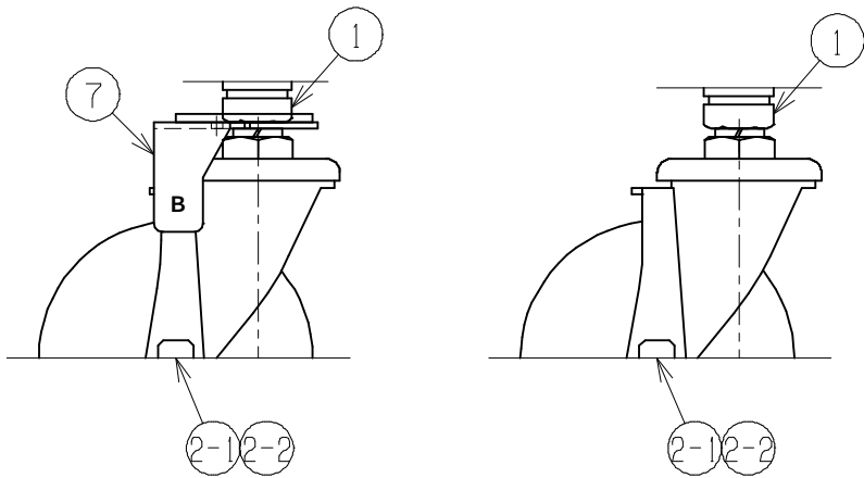
キャスター取付部詳細 尺度1:3
